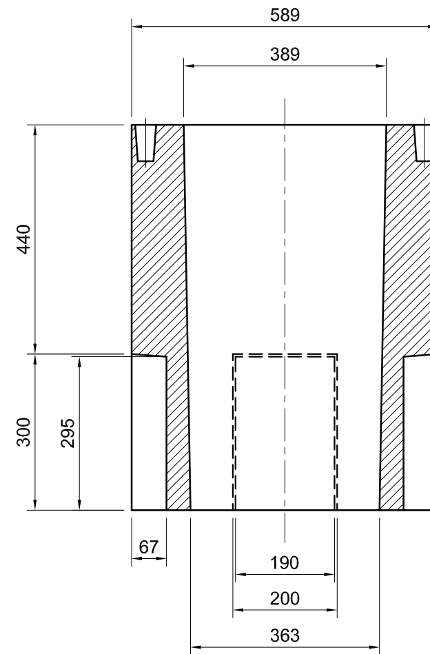
SECCION-B-B
